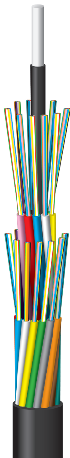
GRHLDV micro FZOMU-SD Micro Ø 5,8 - 10,2 mm Backbonekabel 24 - 288 fibrer
